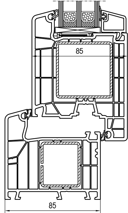
Zugrundeliegende Profil-Kombination für U_f Maßstab: 1:2
